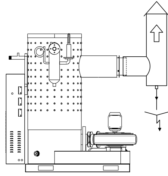
BACA BAĞLANTI DETAYI DETAIL OF CHIMNEY
